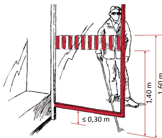
Die auskragende Glaswand ist mit einem Rahmen eingefasst, max. 0,3 m über Boden ertastbar und mit einer lichtundurchlässigen, vorzugsweise weissen Markierung gekennzeichnet.
