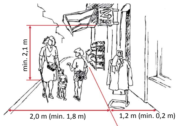
Freie Gehfläche und minimale lichte Höhe
