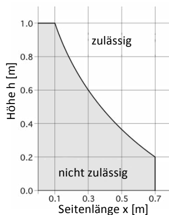
Mindestdimensionen niedriger Hindernisse
