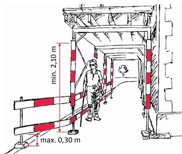
Wegführung und Absicherung von Baugerüsten
